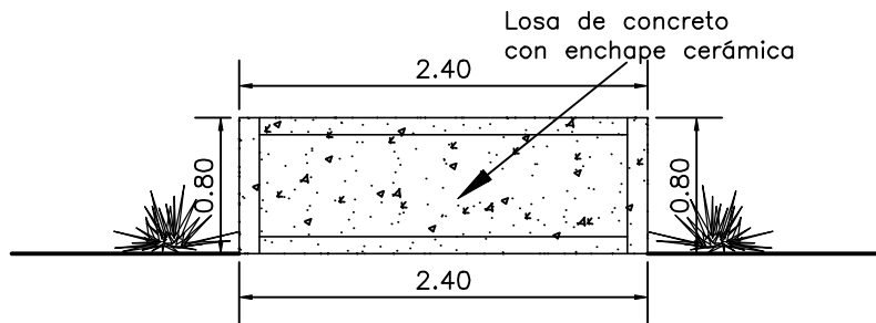
Detalle lateral
