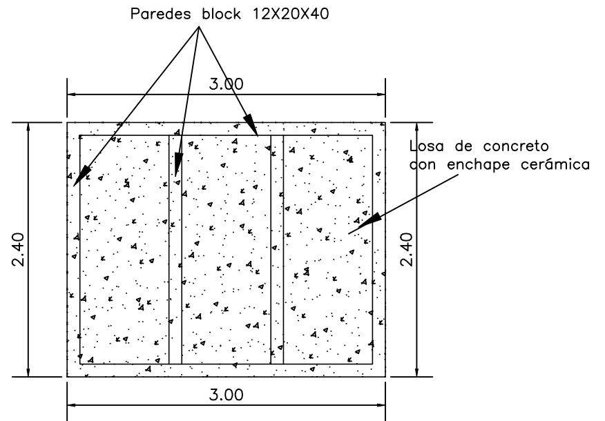
Detalle planta
